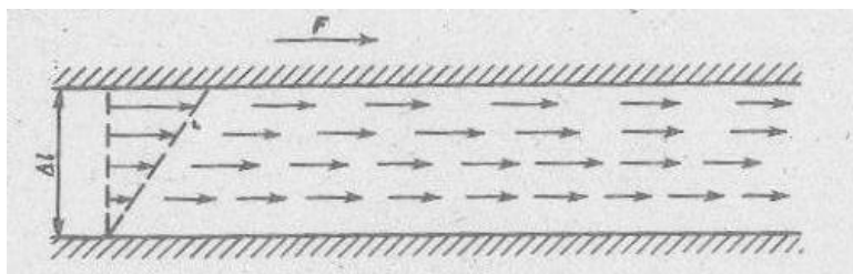
Рис. 1. Визначення в'язкості рідини між двома дотичними пластинами
