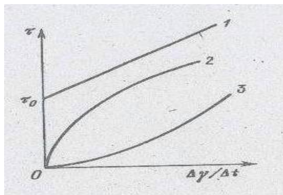
Рис. 4. Реологічна крива не ньютонівських рідин
