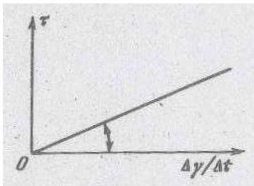
Рис. 3. Реологічна крива ньютонівських рідин
