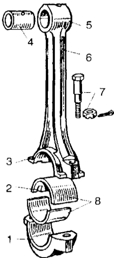
Рис. 2 Шатун:
