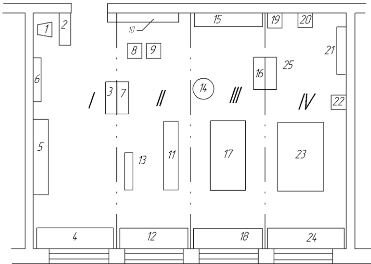
Рис.1.2. Планування слюсарно-монтажної майстерні:
