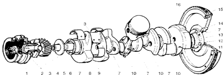
Рис. 3. Колінчастий вал:
