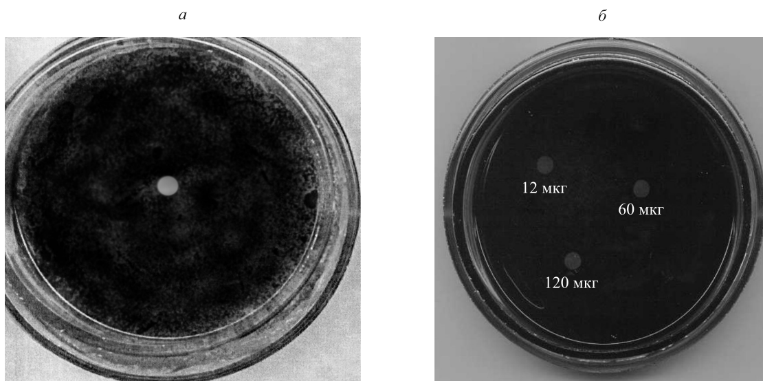
Рис. 2. Чувствительность ассоциативной культуры сульфатовосстанавливающих бактерий: а – к 0,5 % раствору ДМСО (контроль); б – к производным 1–7 (нумерацию см. на рис. 1, в )
