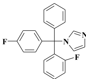
Флутримазол
