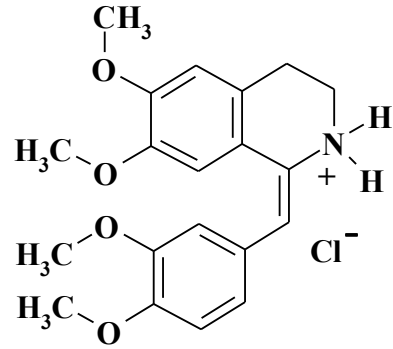
Но-шпа
