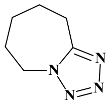
Коразол
