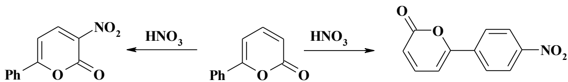
3-Нітро-6-феніл-2H-піран-2-он
