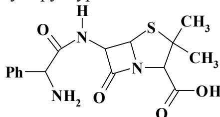
Ампіцилін
