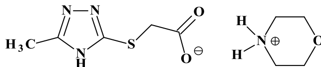
Тіотриазолін
