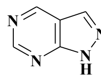
1H-Піразоло[3,4-d]піримідин
