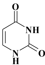
Урацил
