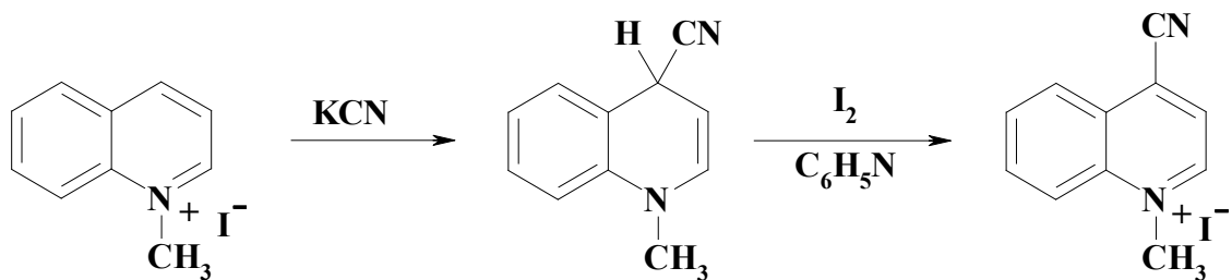
N-Метил-4-ціано-хіноліній йодид
