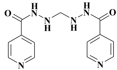
Метазид
