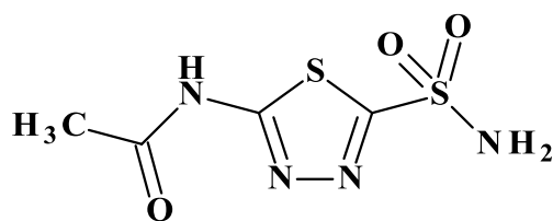
Ацетазоламід
