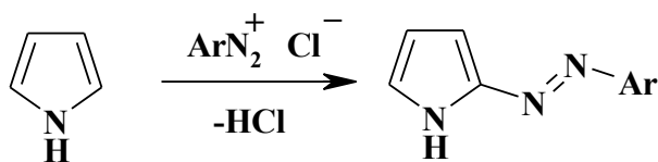
Арилазопірол
