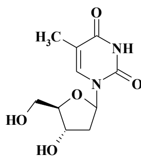
Тимідин
