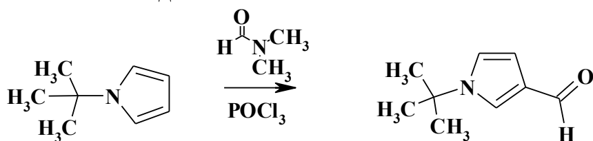
N-Трет-бутил-3-формілпірол
