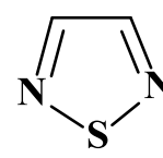
1,2,5-Тіадіазол
