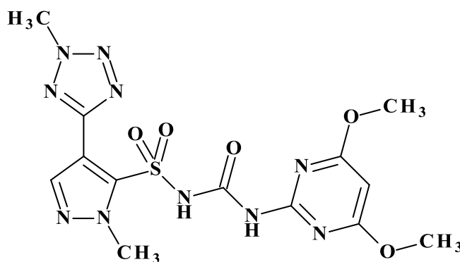
Азімсульфурон
