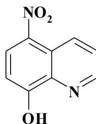
Нітроксолін (5-НОК)
