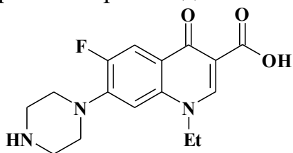
Норфлоксацин
