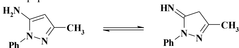
5-Аміно-3-метил-1-фенілпіразол
