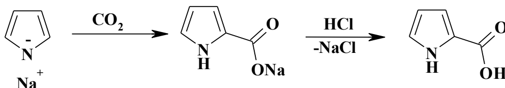
Пірол-2-карбонова кислота
