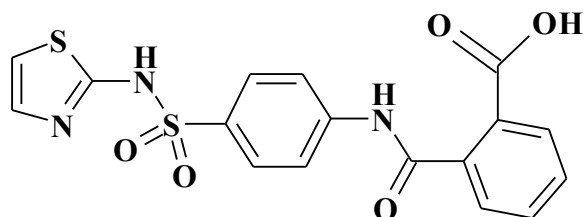
Фталазол
