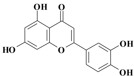
Лутеолін
