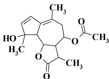
Матрицин
