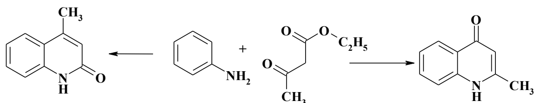
4-Метил-1,2-дигідрохінолін-2-он
