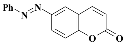
6-Фенілазакумари
