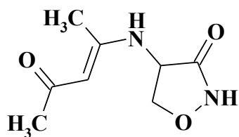
Пентізидон
