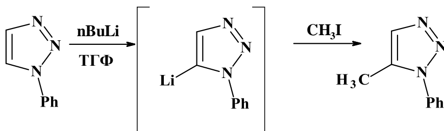
4метил-1-феніл[1,2,3]триазол
