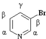
\beta -Бромпіридин
