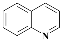
Хінолін
