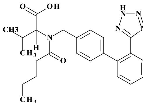
Валсарган
