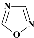
1,2,4-Оксадіазол
