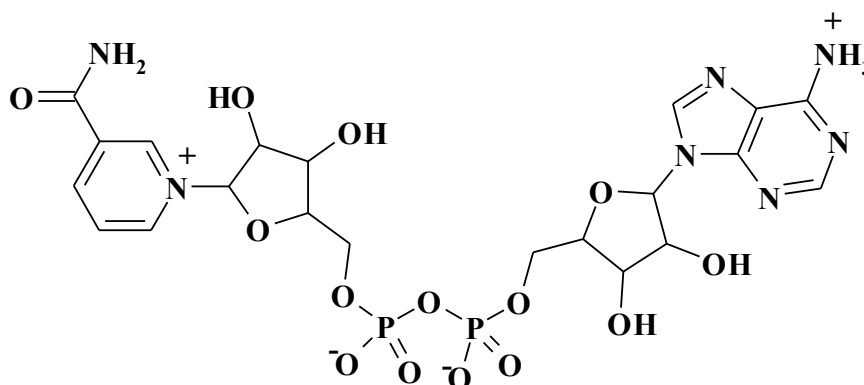
Нікотинамід
