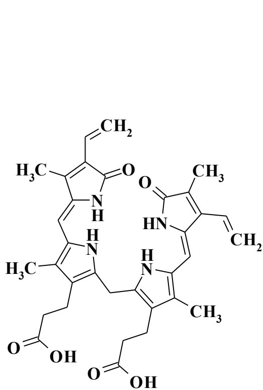
Хлорофіл- \alpha
