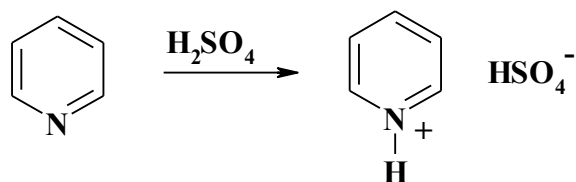
Піридиній гідросульфат
