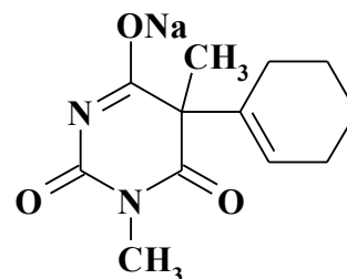
Гексенал
